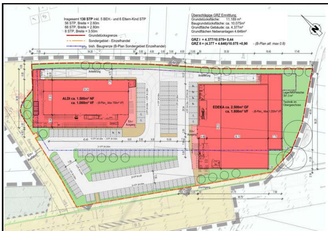
Abb. 2: Planzeichnung mit Grundriss der neuen Gebäudehallen von Aldi und Edeka am Fliederweg
