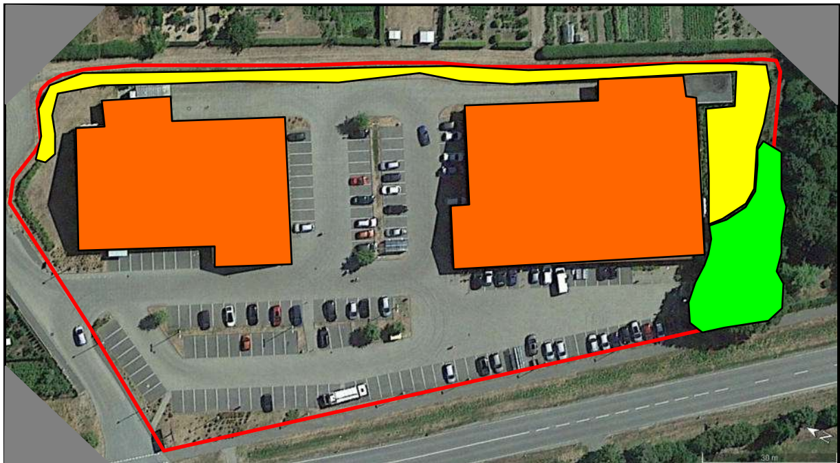
Abb. 5: Darstellung der Lebensräume der drei festgestellten Habitatgilden „Siedlungsarten“ (orange), Strauch-Unterholzarten (gelb) und Baum-Unterholzarten (grün)
