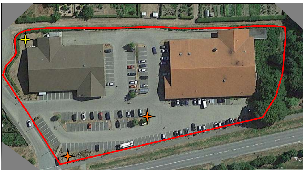
Abb. 15: Lage der Magerrasenfragmente mit den beiden nach Bundesartenschutzverordnung geschützten Pflanzenarten; gelber Stern: Lage Sand-Strohblume ( Helichrysum arenarium ), ca. 120 Exemplare, oranger Stern: Lage Sand-Grasnelke ( Armeria maritima ssp. elongata ), jeweils mehrere Einzelexemplare
